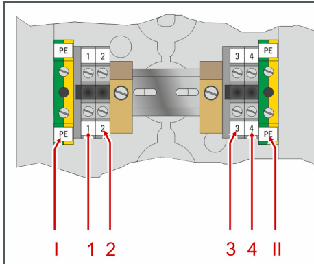
Anschluss – Gerätedeckel-Innenseite
