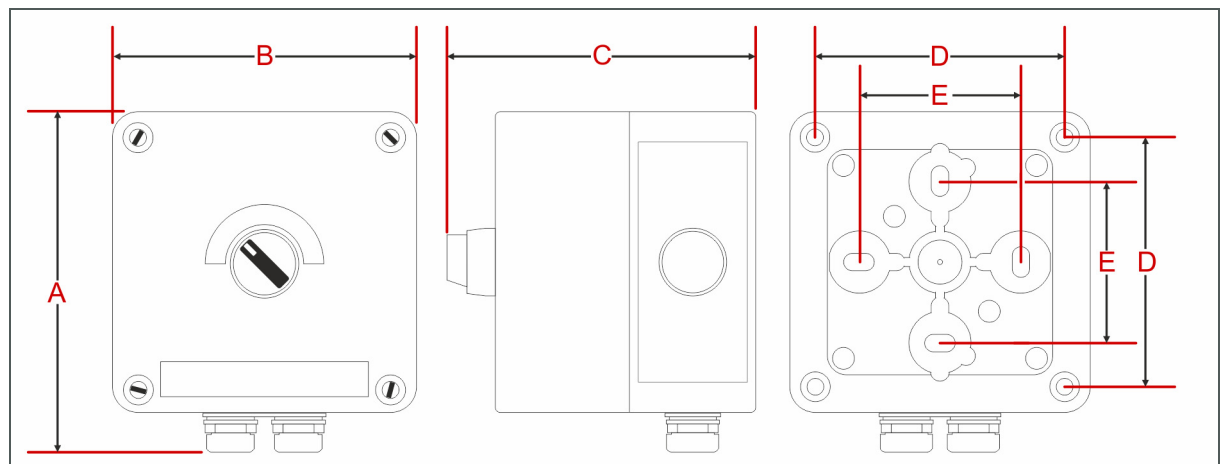
Abmessungen
