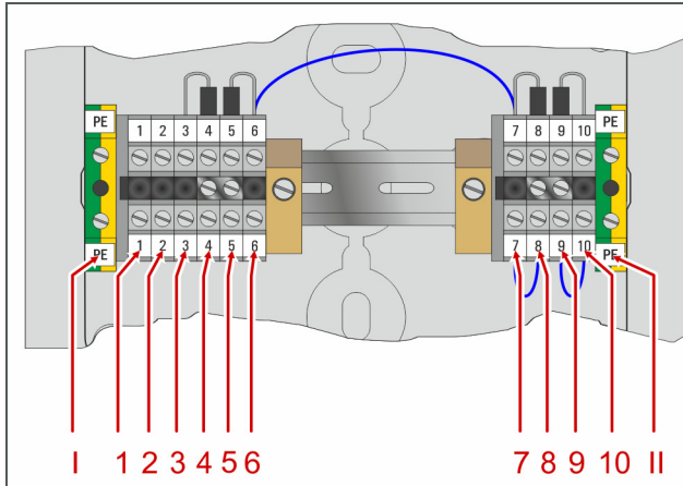
Anschluss – Gerätedeckel-Innenseite
